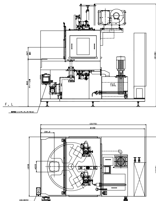
■ 寸法図 (KTI-1000)
