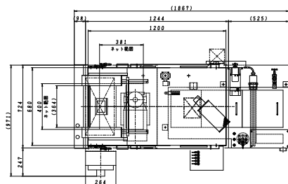
■ 寸法図 (SPC-102-B)
