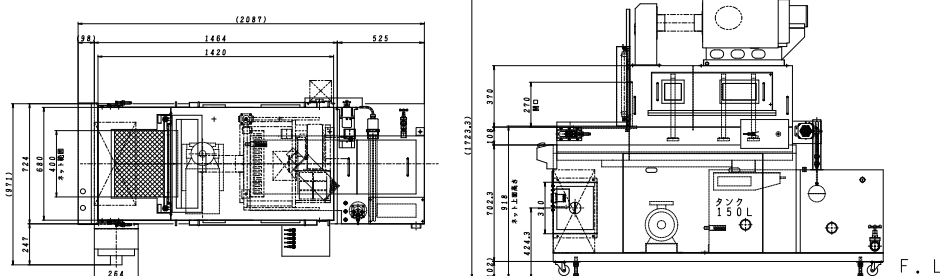
■寸法図 (SPC-203-B)
