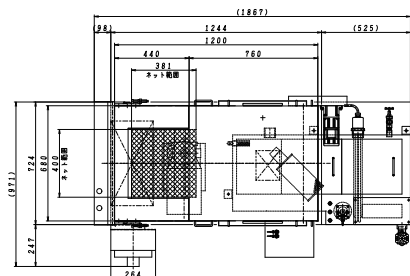
■ 寸法図 (SPC-101-B)
